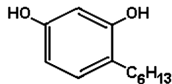
4- n -hexylresorcinol
