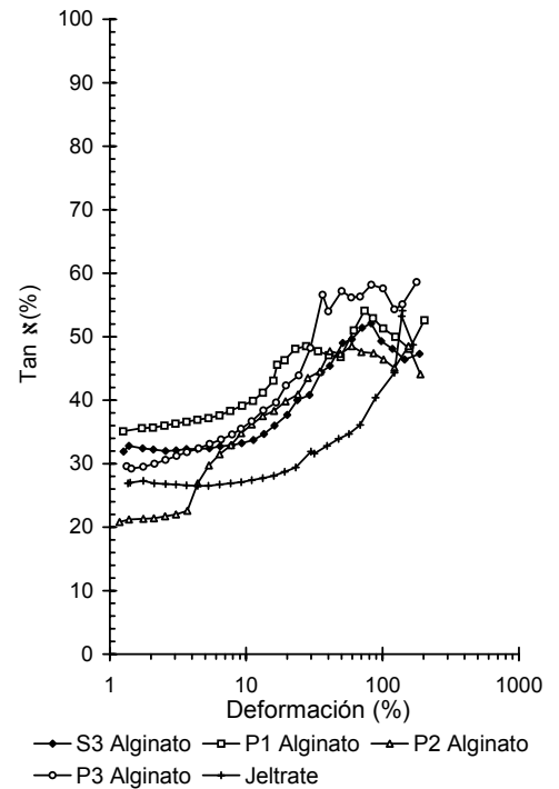
Figure 4. Loss factors of alginate dental impression material produced with the a5 formulation. Figura 4. Factores de pérdida del material para impresión dental producido con alginatos y la formulación a5.
