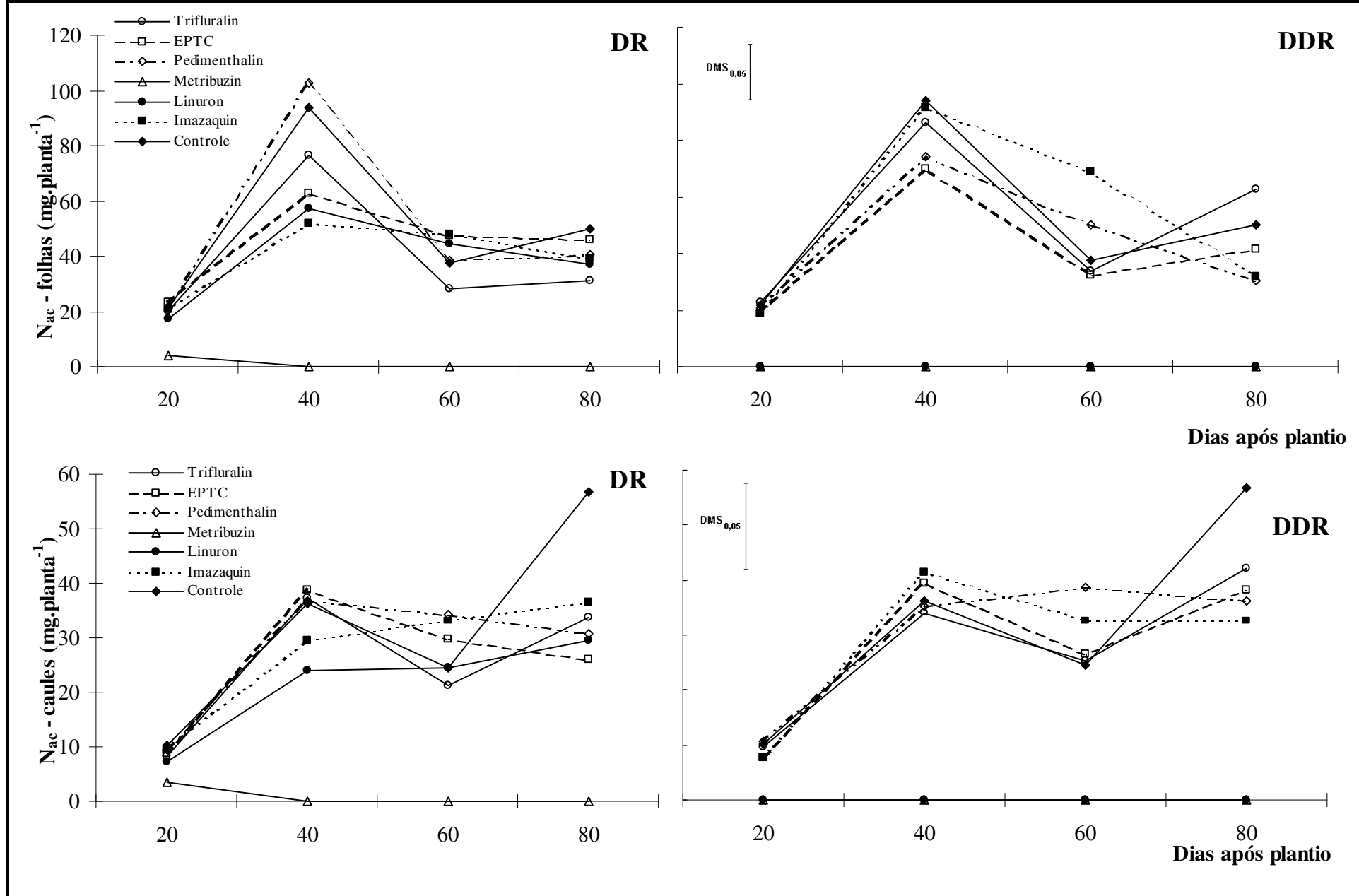
FIG. 1. Andamento seguido na acumulação de nitrogênio ( N_{ac} ) total nas folhas e caules das plantas da cultivar de caupi BR-IPA-206, infectadas com Bradyrhizobium NFB 09, em diferentes tratamentos estabelecidos (média de 3 repetições; DR = dose recomendada; DDR = dobro da dose recomendada).
